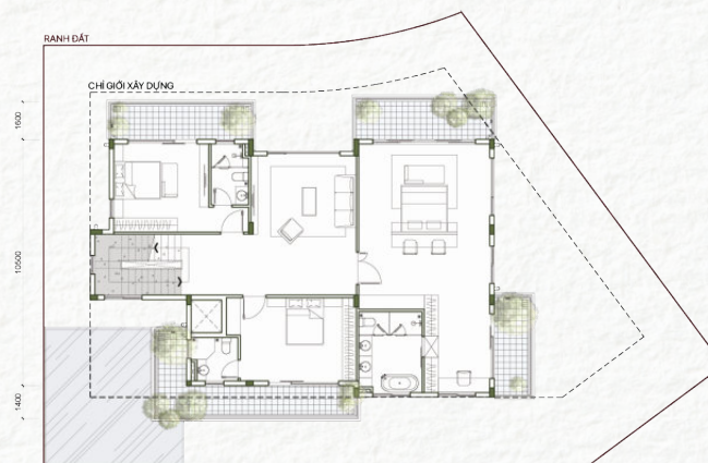
Tầng 02
