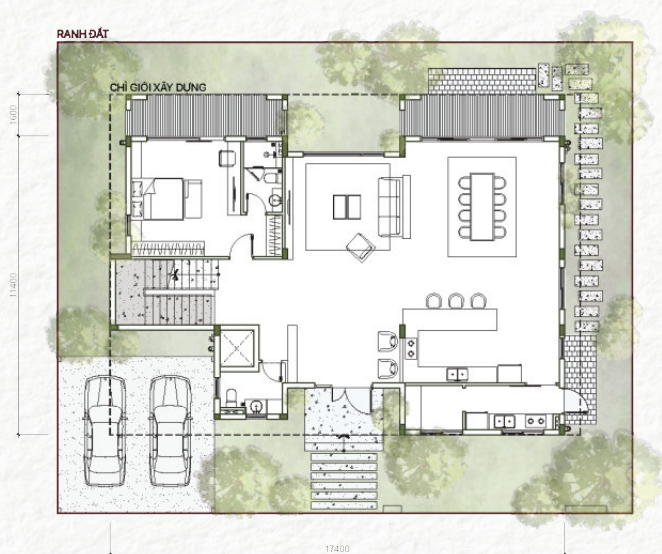
Tầng 01
