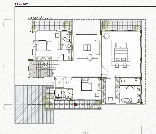
Tầng 02
