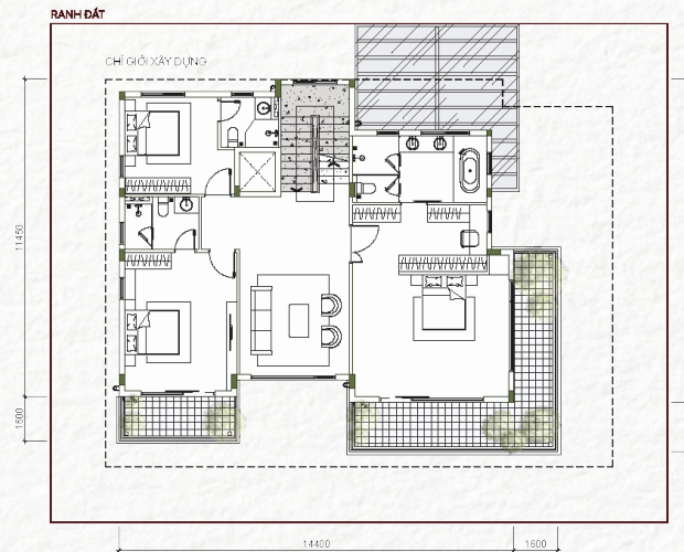
Tầng 02
