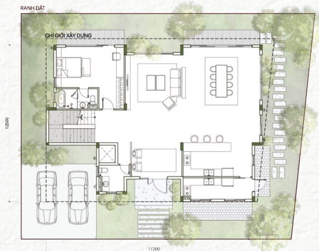
Tầng 01
