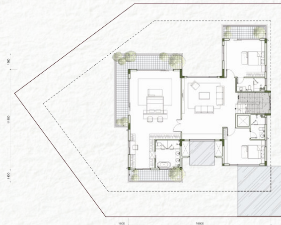
Tầng 02
