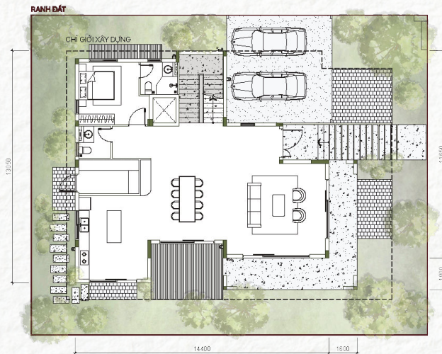
Tầng 01
