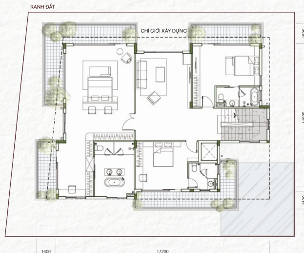
Tầng 02
