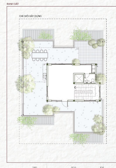
Tầng 03
