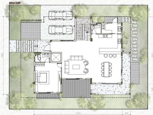
Tầng 01
