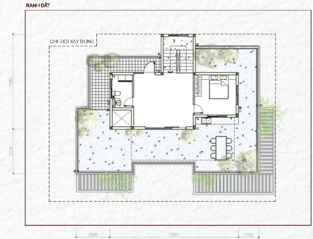
Tầng 03
