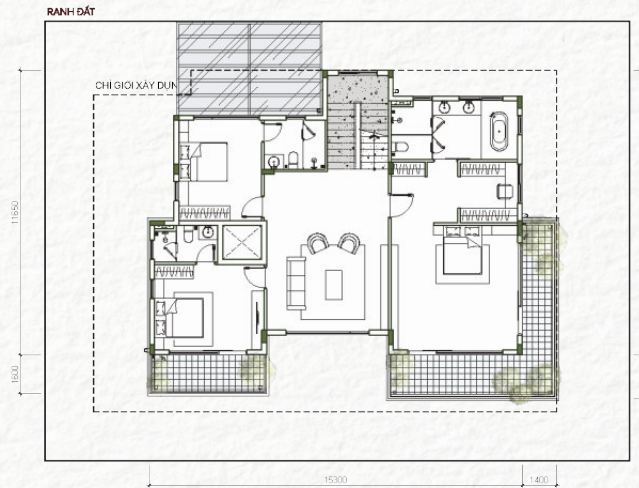
Tầng 02
