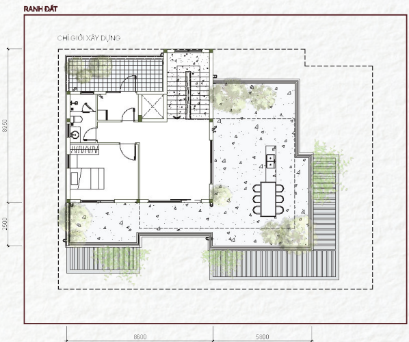
Tầng 03
