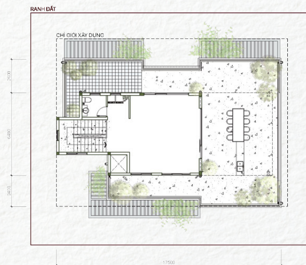
Tầng 03
