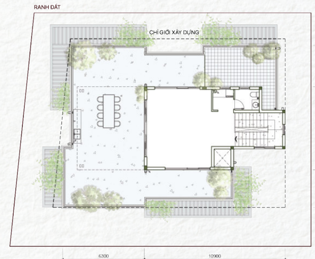
Tầng 03
