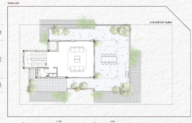
Tầng 03
