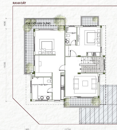
Tầng 02
