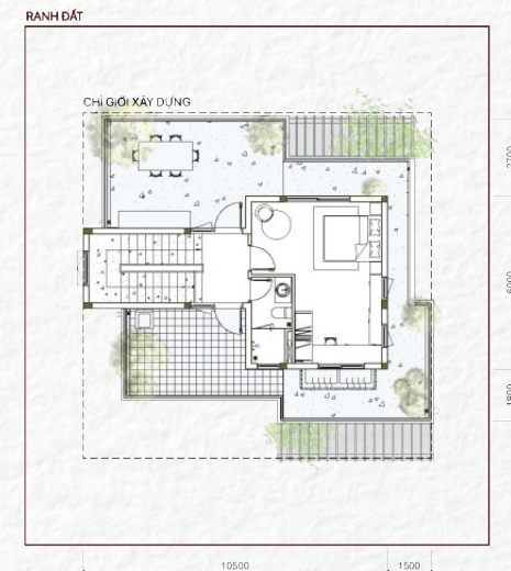
Tầng 03
