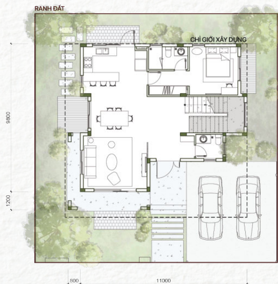
Tầng 01
