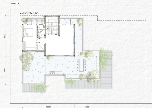
Tầng 03
