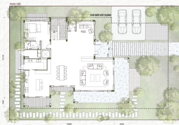
Tầng 01
