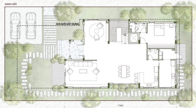
Tầng 01
