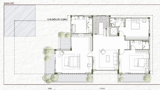
Tầng 02
