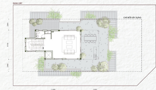
Tầng 03
