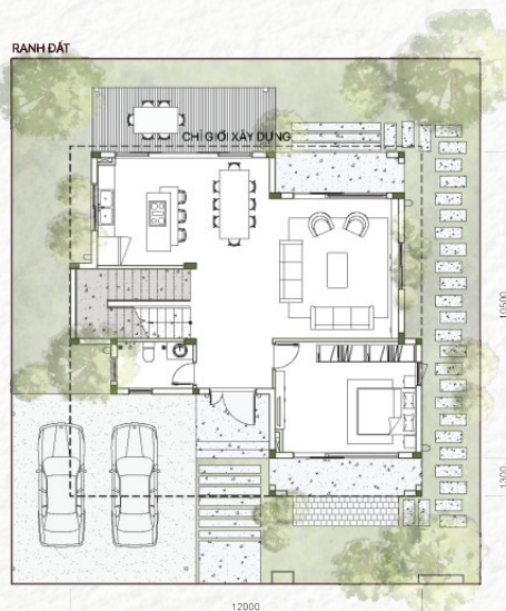
Tầng 01
