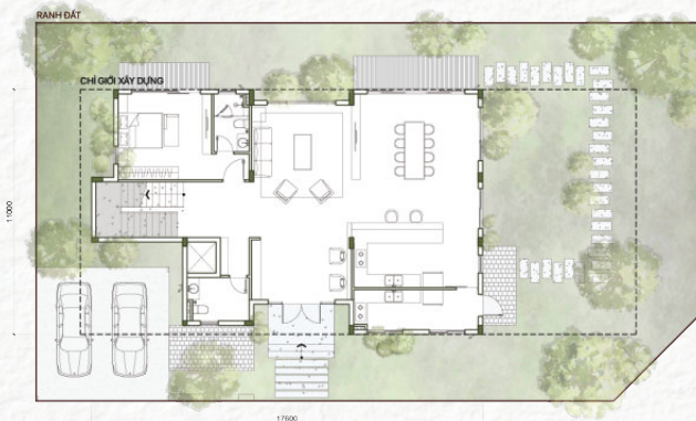
Tầng 01
