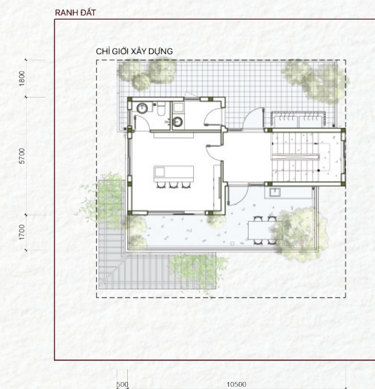
Tầng 03
