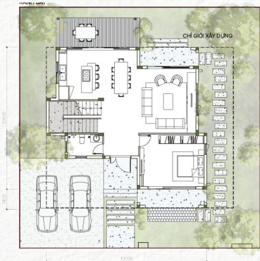
Tầng 01
