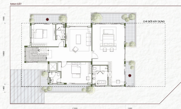
Tầng 02
